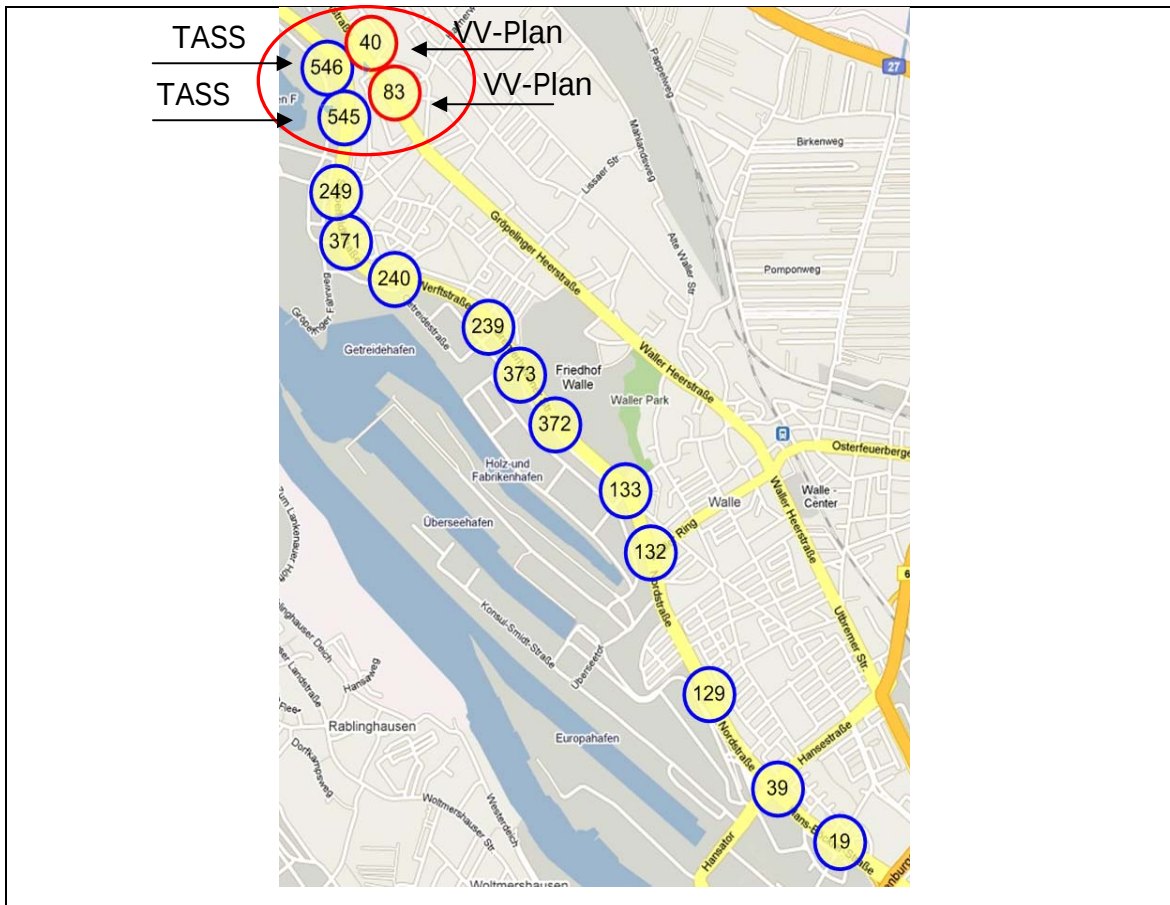
Bild 9: Übersichtsplan TASS Hafenrandstraße Süd
